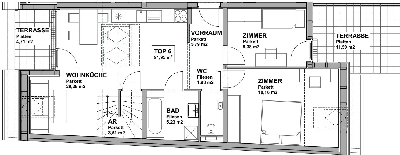
GRUNDRISS DACHGESCHOSS M 1:100
