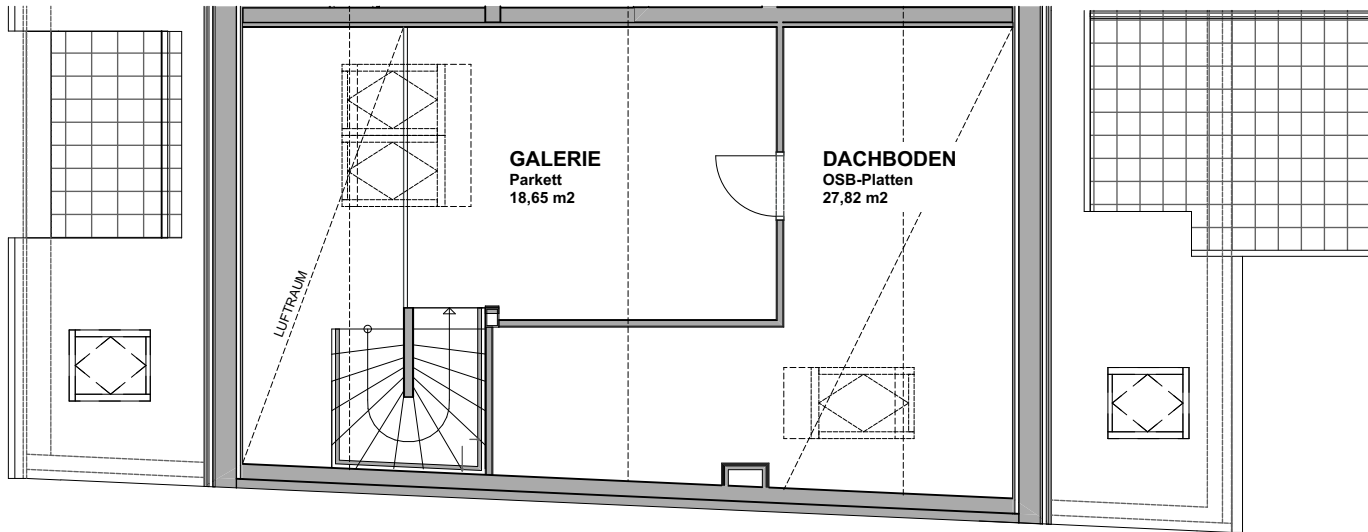
GRUNDRISS GALERIE M 1:100
