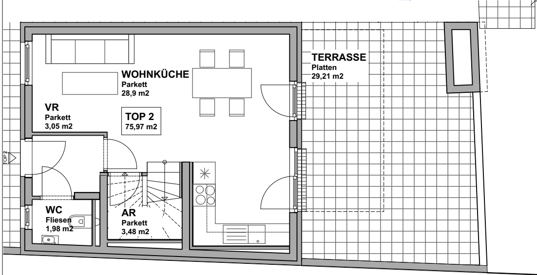
GRUNDRISS ERDGESCHOSS M 1:100
