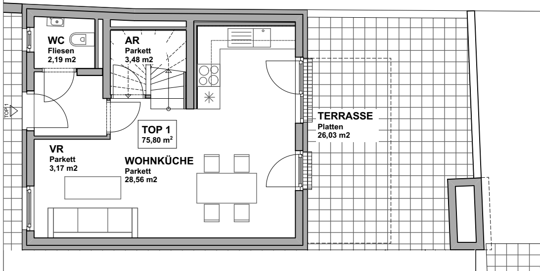
GRUNDRISS ERDGESCHOSS M 1:100
