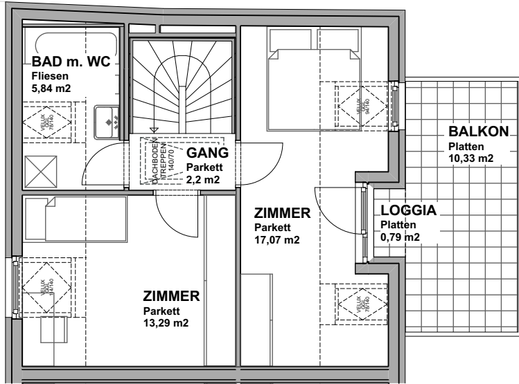
GRUNDRISS DACHGESCHOSS M 1:100
